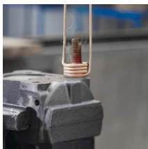
Sugriuvusių varžtų išsukimas
