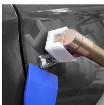
Transporto priemonės identifikacinių plokštelių nuėmimas
